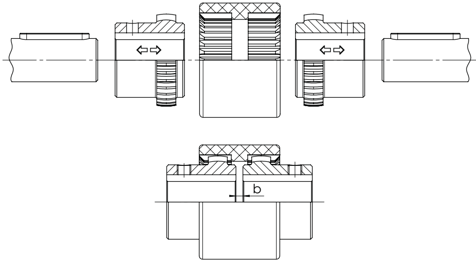
Figura 4-2 - SITEX®: montaggio
