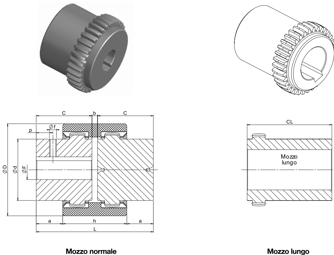
Figura 2-1 - Mozzi SITEX®
