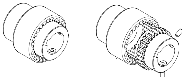
Figura 4-3 - Giunto SITEX® Nylex esecuzione CV
